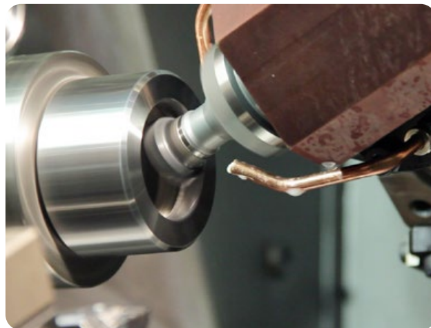
Prozesssicher und präzise: In Kombination mit hochwertigen Werkzeugen und passenden Aufnahmen erschließt Wedco auch anspruchsvolle Dreh-Fräs-Kombinationen – wie etwa das Power Skiving – für eine wirtschaftliche Fertigung.
