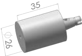
Drehhalter Rohling Ø 26 Turning holder blank Ø 26
