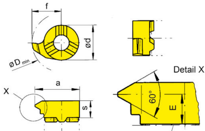
Klemmhalter Stirnseite
